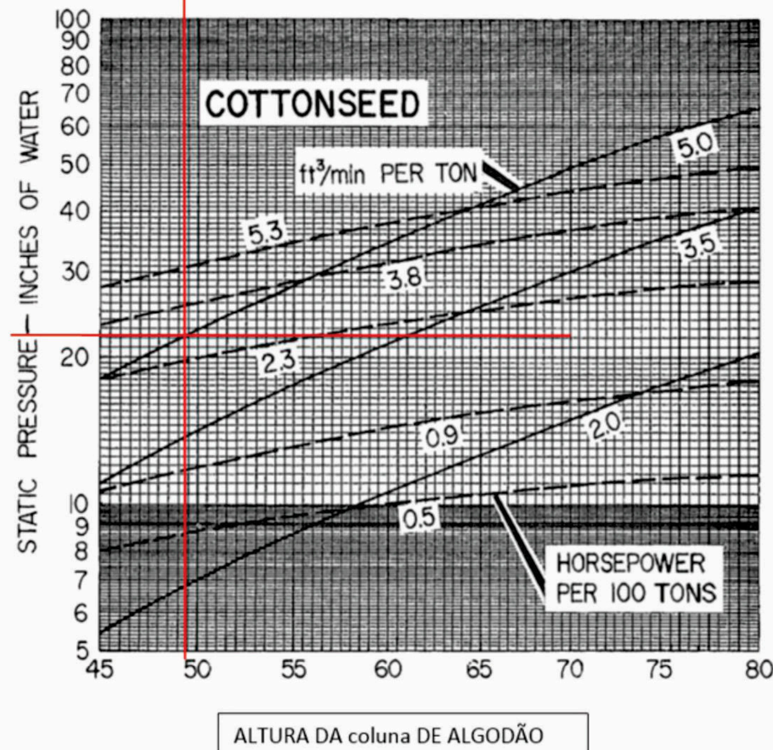
Figura 28. Requisitos de potência do ventilador para aeração de algodão e pressão estática desenvolvidos em diferentes taxas de fluxo de ar, em profundidades de algodão variando de 45 a 80 pés.
